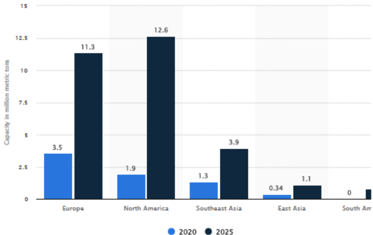
Abb. 4 Weltweite HVO-Produktionskapazität 2020, Prognose für 2025 5
