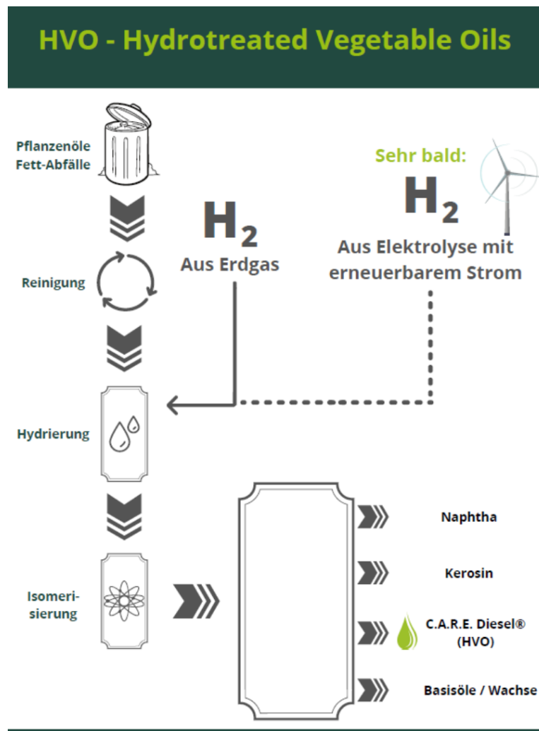
Abb.2: Herstellung von HVO 3
