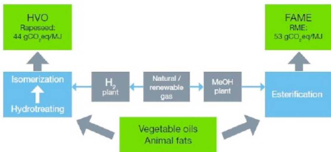
Abb1. Vergleich der CO 2 -Emissionen von HVO und Biodiesel (RME) 2 (bei Hydrierung mit grauem Wasserstoff bzw. Umesterung mit grauem Methanol)
