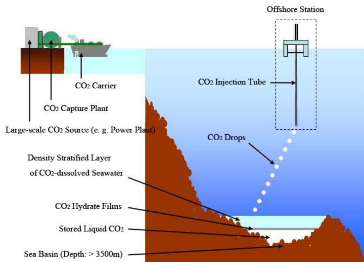
Abb.7 CO 2 -Tiefenverpressung im Meer 14
