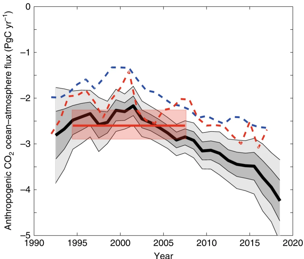
Abb. 3 Entwicklung der anthropogenen CO 2 -Aufnahme bis 2018 auf Basis verschiedener Rechenmodelle 5 (1 Petagramm Kohlenstoff entspricht 1 Gigatonne Kohlenstoff oder 3,66 Gigatonnen CO 2 )
