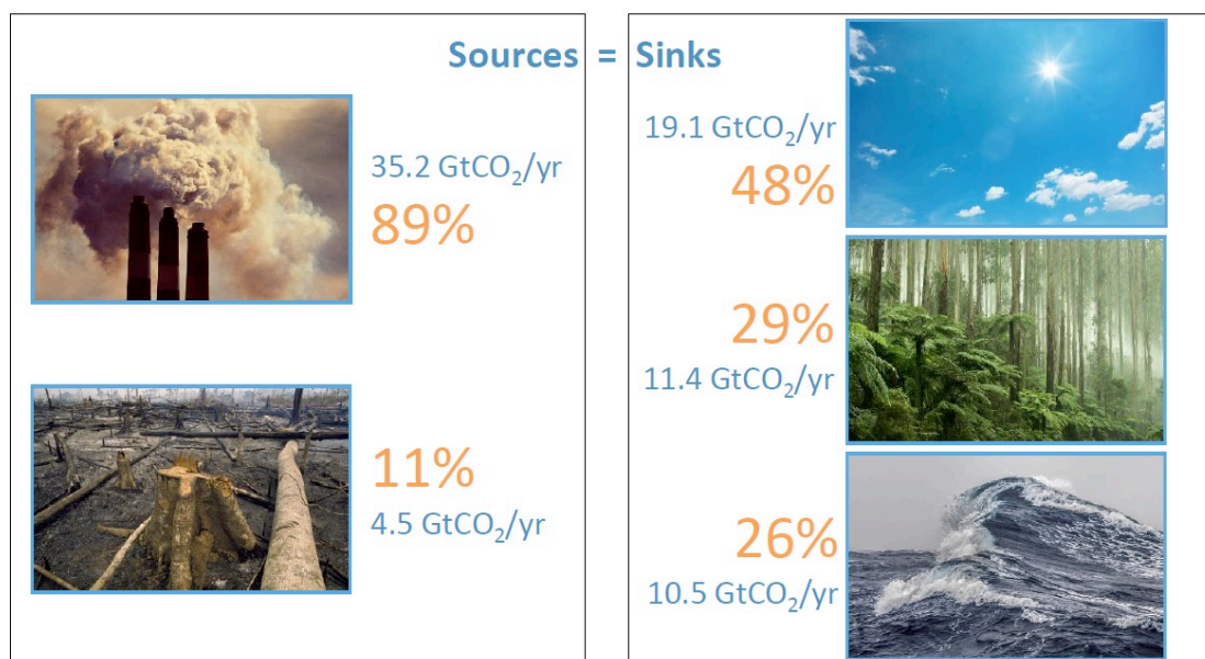
Abb. 8 Bilanz der globalen CO 2 -Emission und -Aufnahme im Jahresdurchschnitt 2012 - 20212
